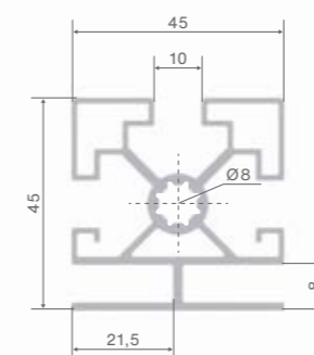
ZWISCHENPROFIL 45 x 45
