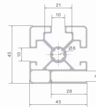
RAHMENPROFIL 45 x 45
