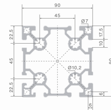
STREBENPROFIL 90 x 90
